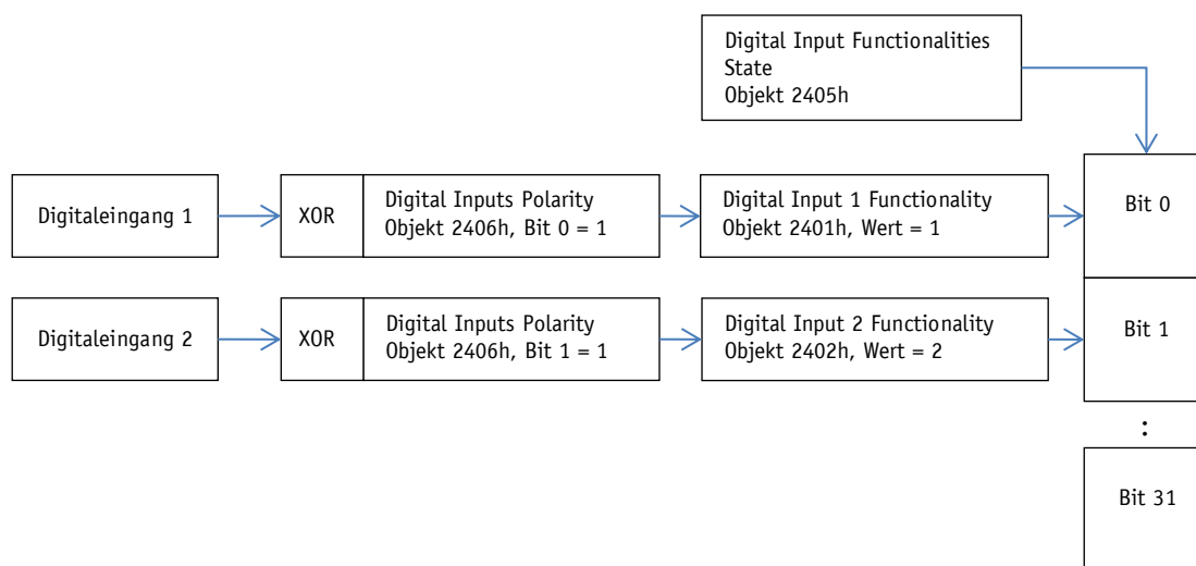
Abb. 10: Beispielkonfiguration Endschalter
