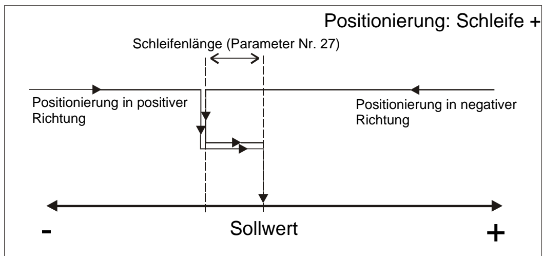
Abb. 3: Positionierung Schleife+
