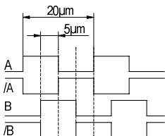
Abb. 2: Ausgabe der Quadratursignale
