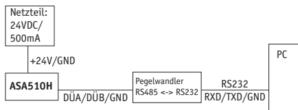
Abb. 3: Blockschaltbild RS485-Verbindung
