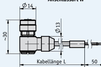
Anschlussart W
