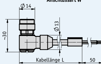
Anschlussart W
