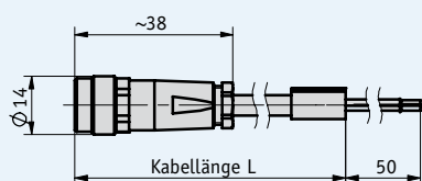
Anschlussart GE
