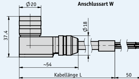
Anschlussart W
