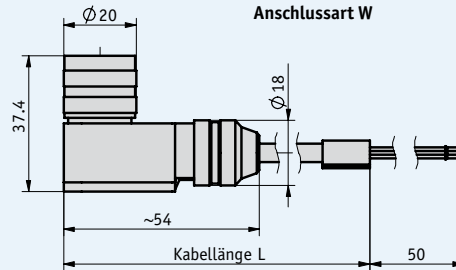
Anschlussart W
