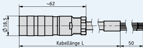
Anschlussart GE
