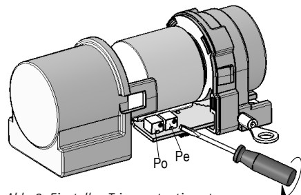
Abb. 8: Einstellen Trimpotentiometer
