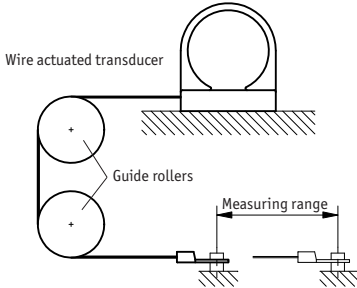
Fig. 3: Guide roller
