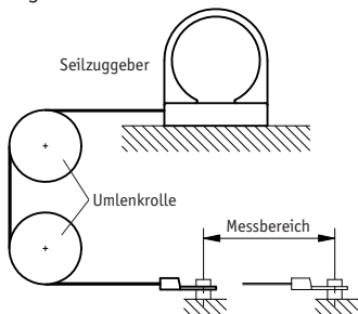
Abb. 3: Umlenkrolle
