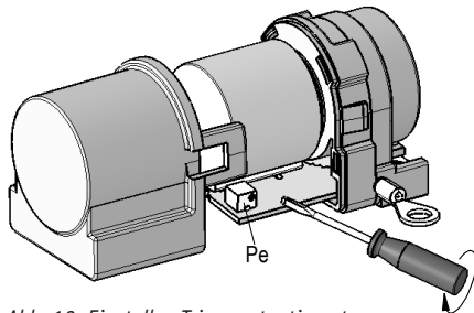
Abb. 10: Einstellen Trimpotentiometer
